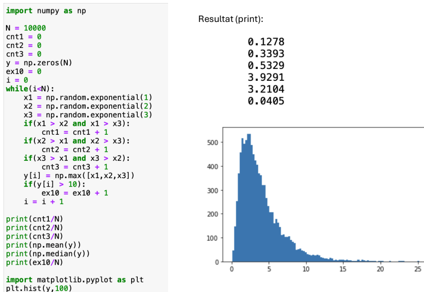
Figur 2: Monte Carlo simulering av levetider for tre lyspærer. Pythonkode (venstre) og resultat av koden (høyre).
